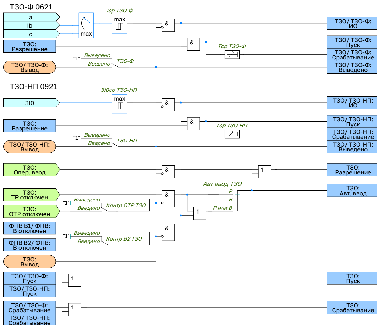
Рисунок 2.31 – Функциональная схема логики ТЗО
