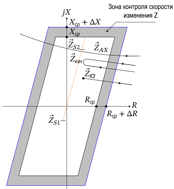
Рисунок 2.15 – Характеристики реле сопротивления, используемые для блокировки при качаниях по скорости изменения сопротивления
