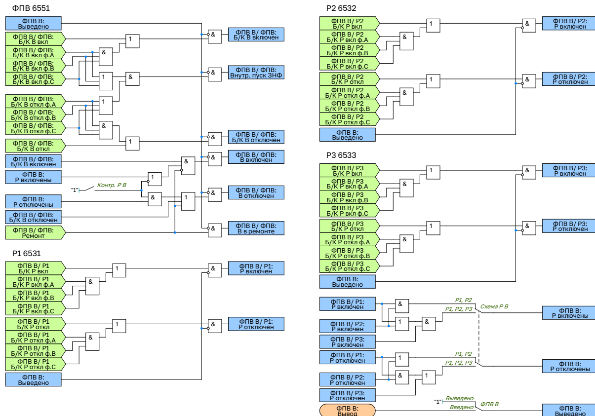
Рисунок 2.45 – Функциональная схема логики ФПВ В1
